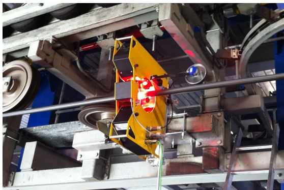
Premiers contrôles visuels très concluants à l'aide du système Winspect, ici câble 45 mm sur le télécabine Médran 1.
